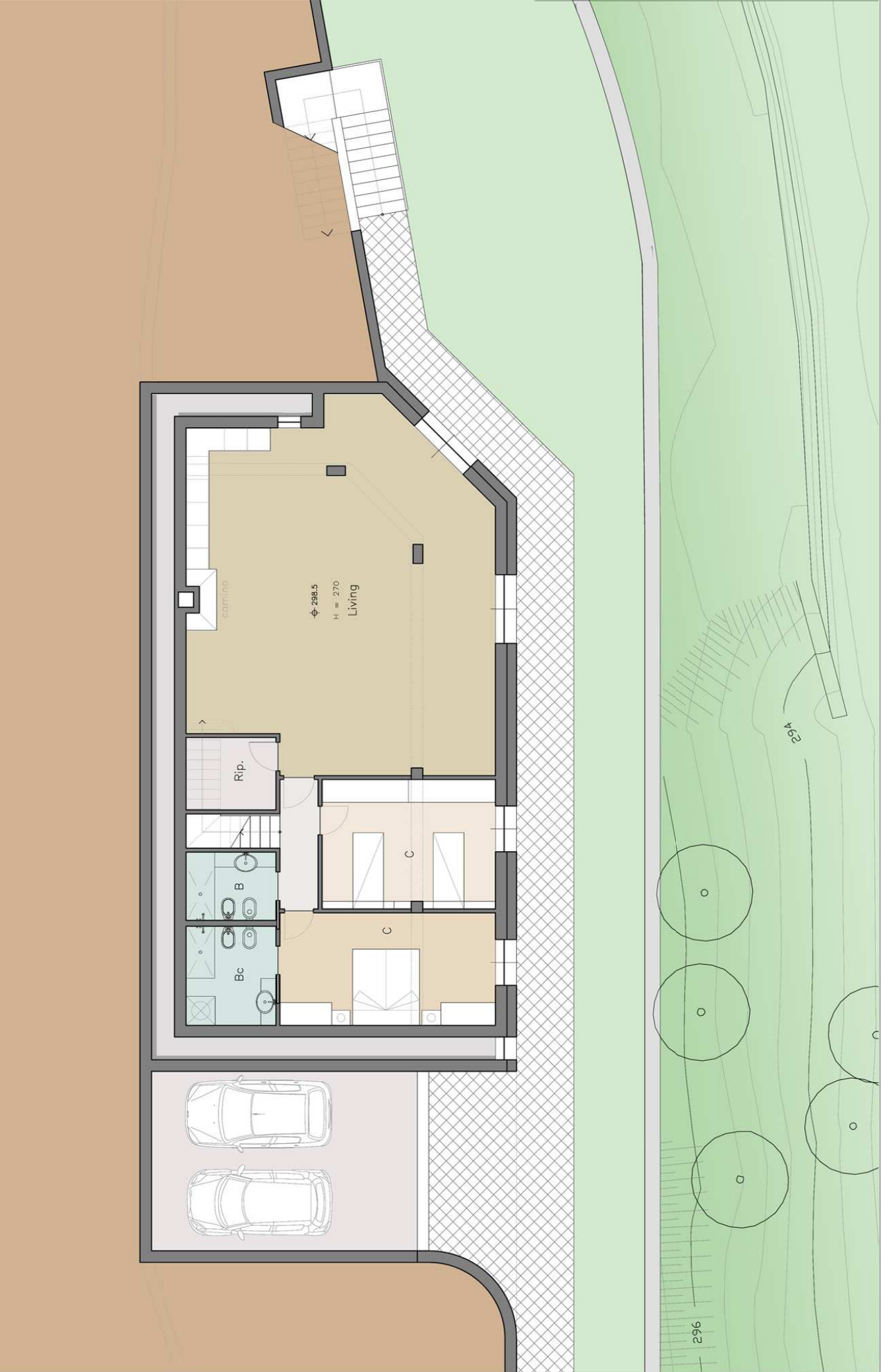
PLANIMETRIA LIVELLO GIARDINO
